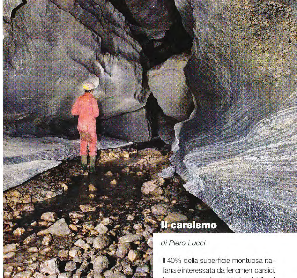
Un meandro nella Grotta Risorgente del Rio Basino (foto P. Lucci).
