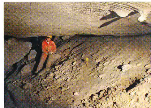
Riempimenti in un ramo fossile del sistema Stella-Basino (foto P. Lucci).
