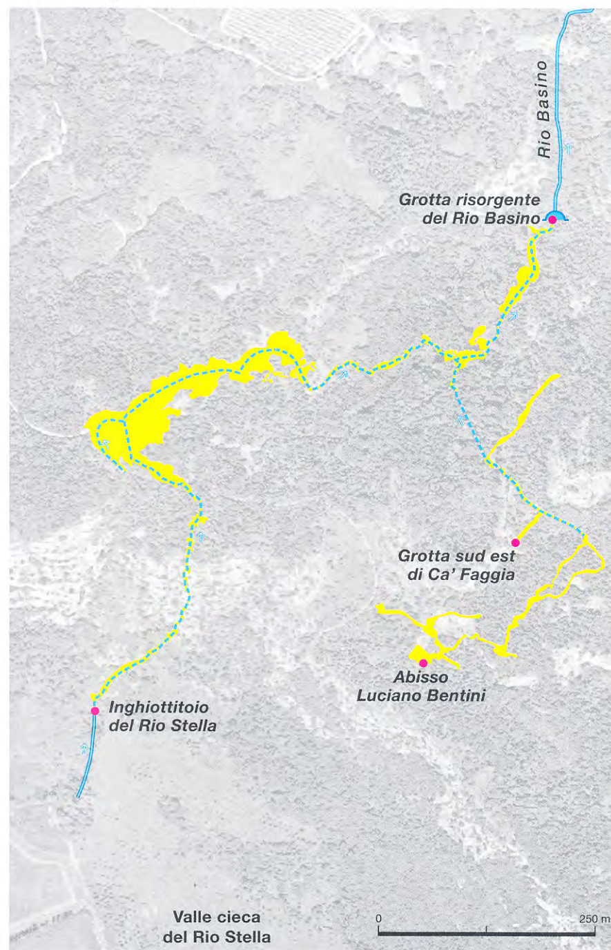
Il sistema carsico "Inghiottitoio del Rio Stella-Grotta Risorgente del Rio Basino-Abisso Luciano Bentini".
