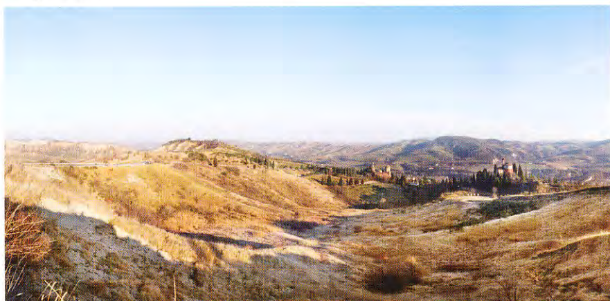
La valle cieca della Volpe. A destra il Santuario del Monticino, a sinistra la Rocca e la Torre dell'Orologio (foto P. Lucci).
