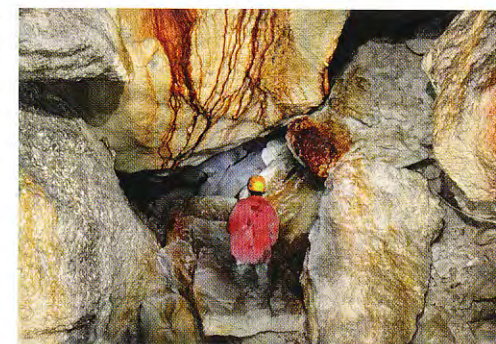
Frana nella prima parte del percorso sotterraneo del Rio Stella. Da notare, sopra lo speleologo, una colata calcarea: il colore rosso-bruno è in relazione al contenuto di acidi organici provenienti dal soprastante terreno (foto P. Lucci).
